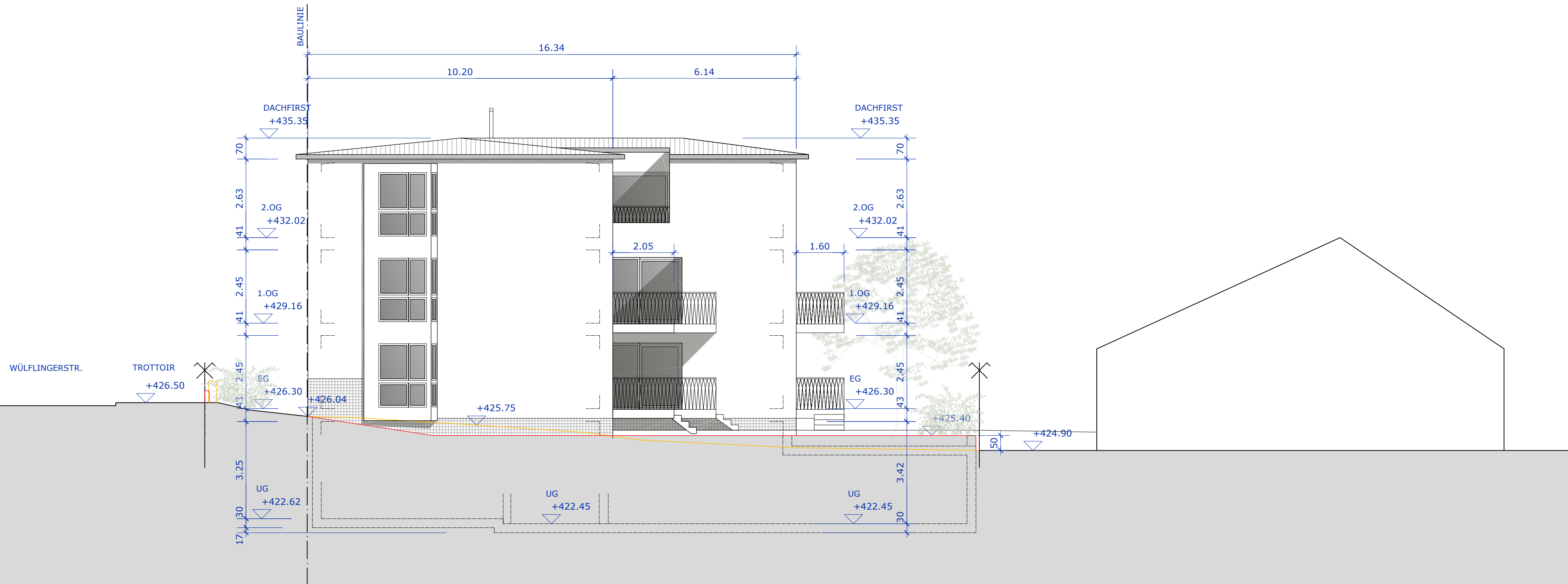
FASSADE NORDWEST
