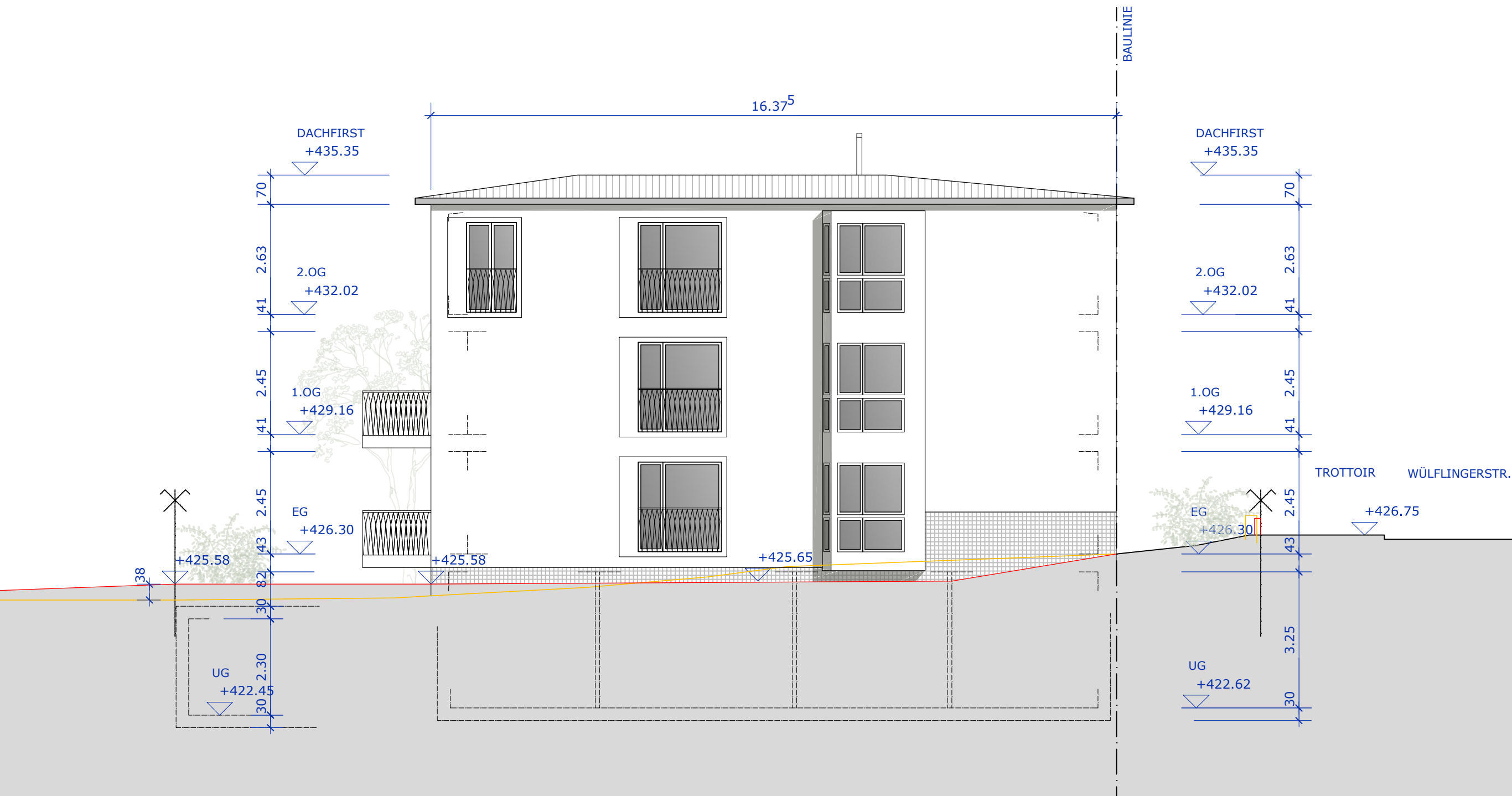
FASSADE SÜDOST
