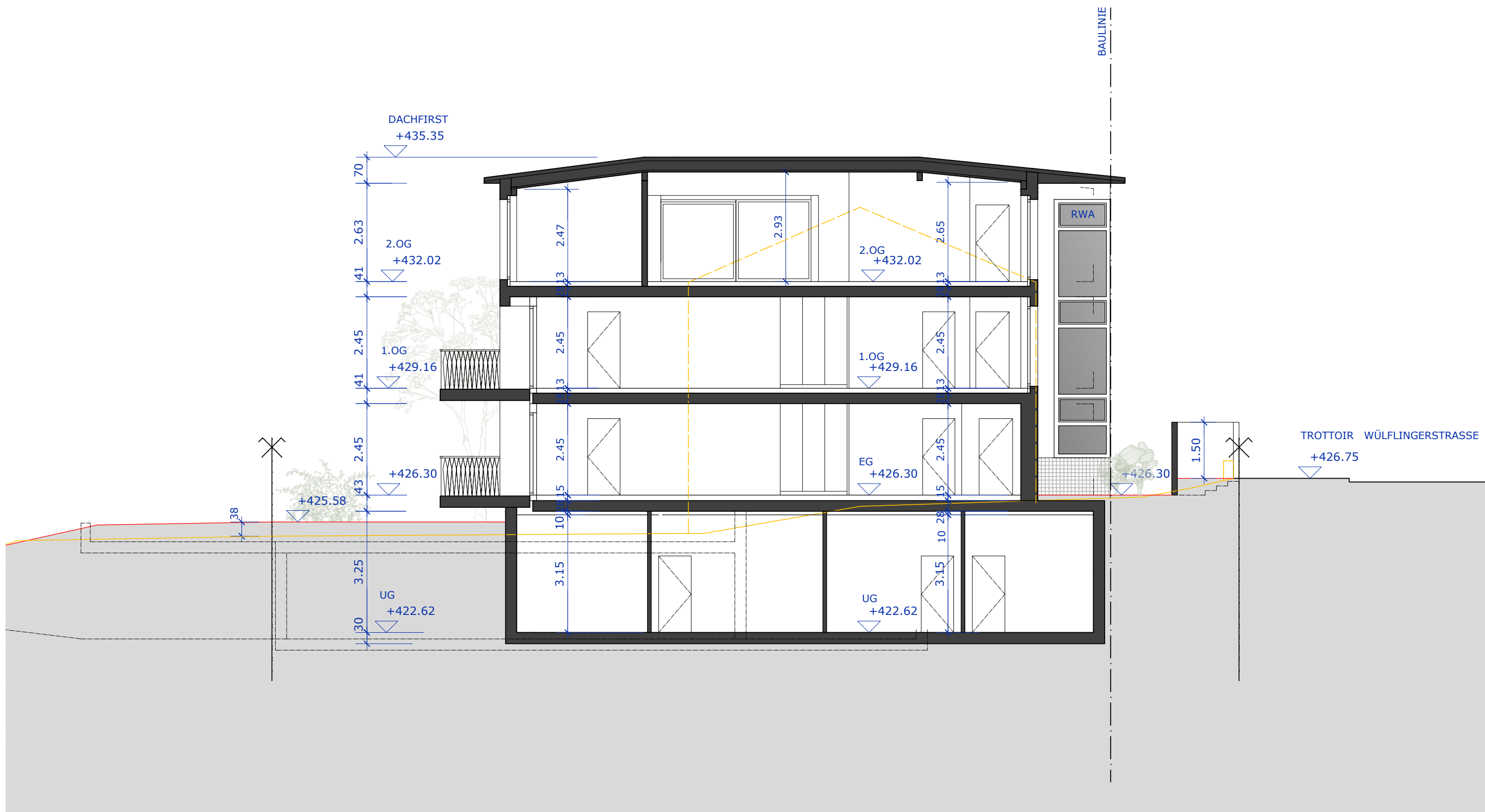
SCHNITT A-A
