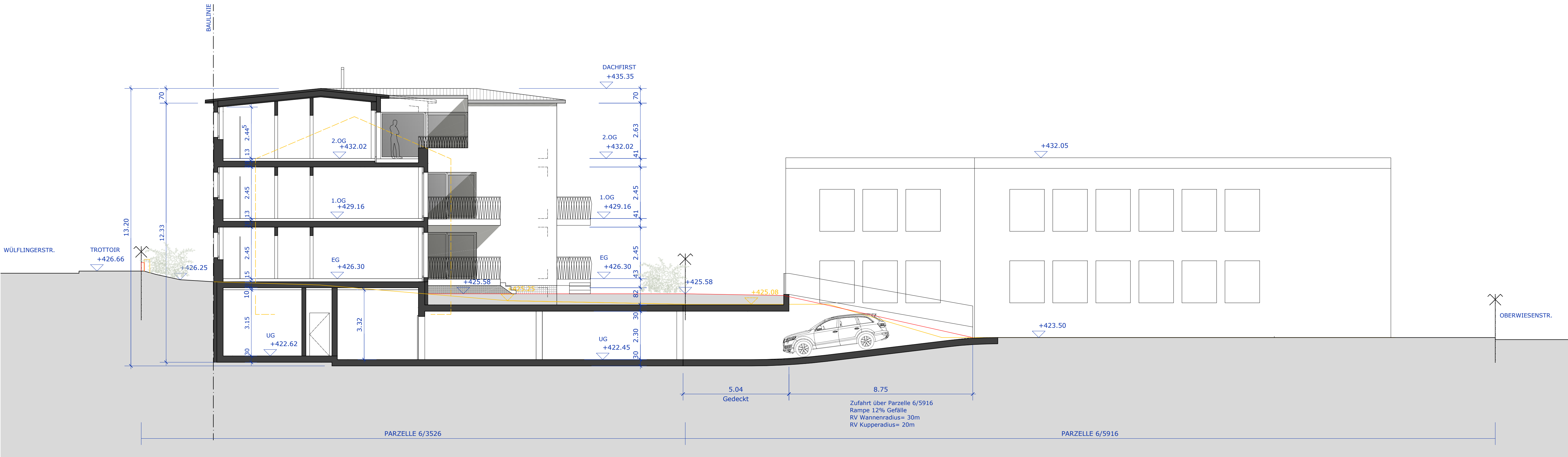
SCHNITT B-B
