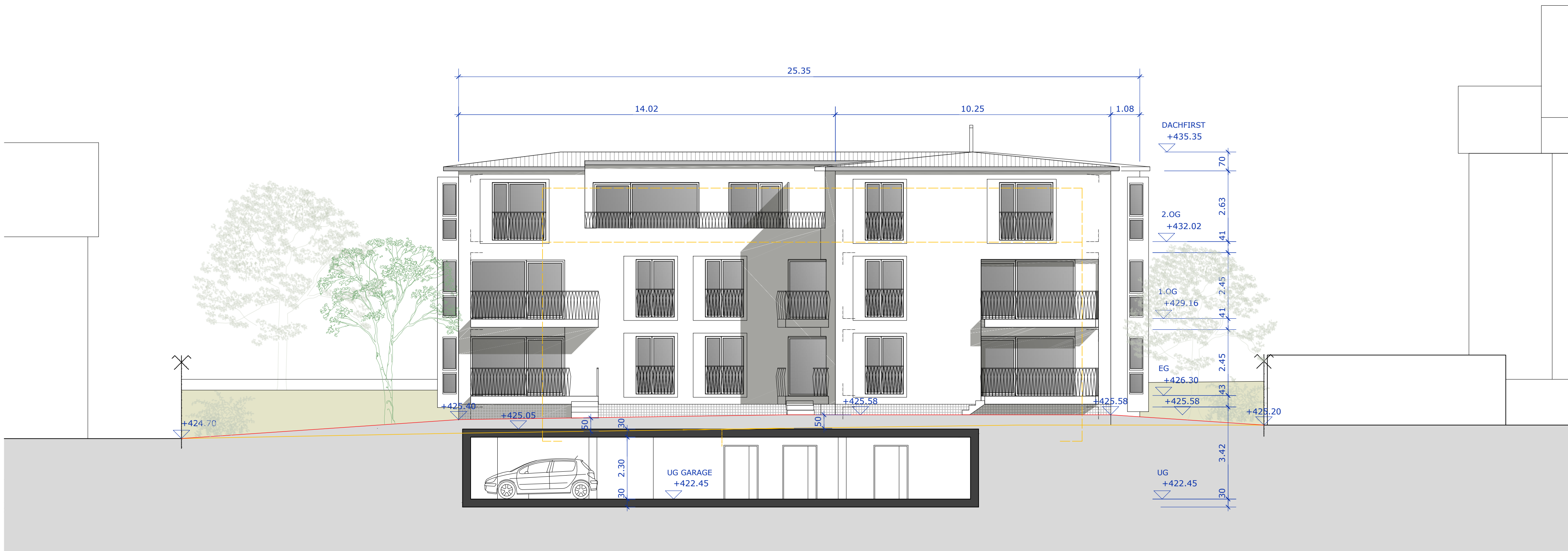
FASSADE SÜDWEST / SCHNITT C-C
