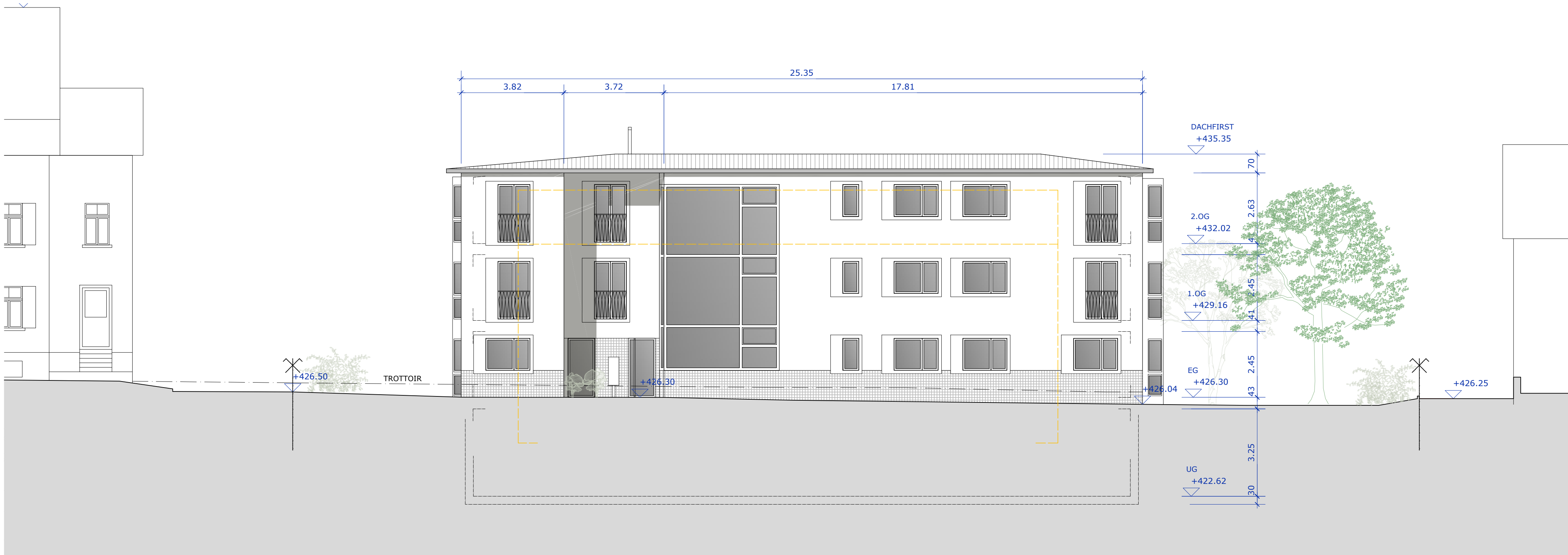
FASSADE NORDOST
