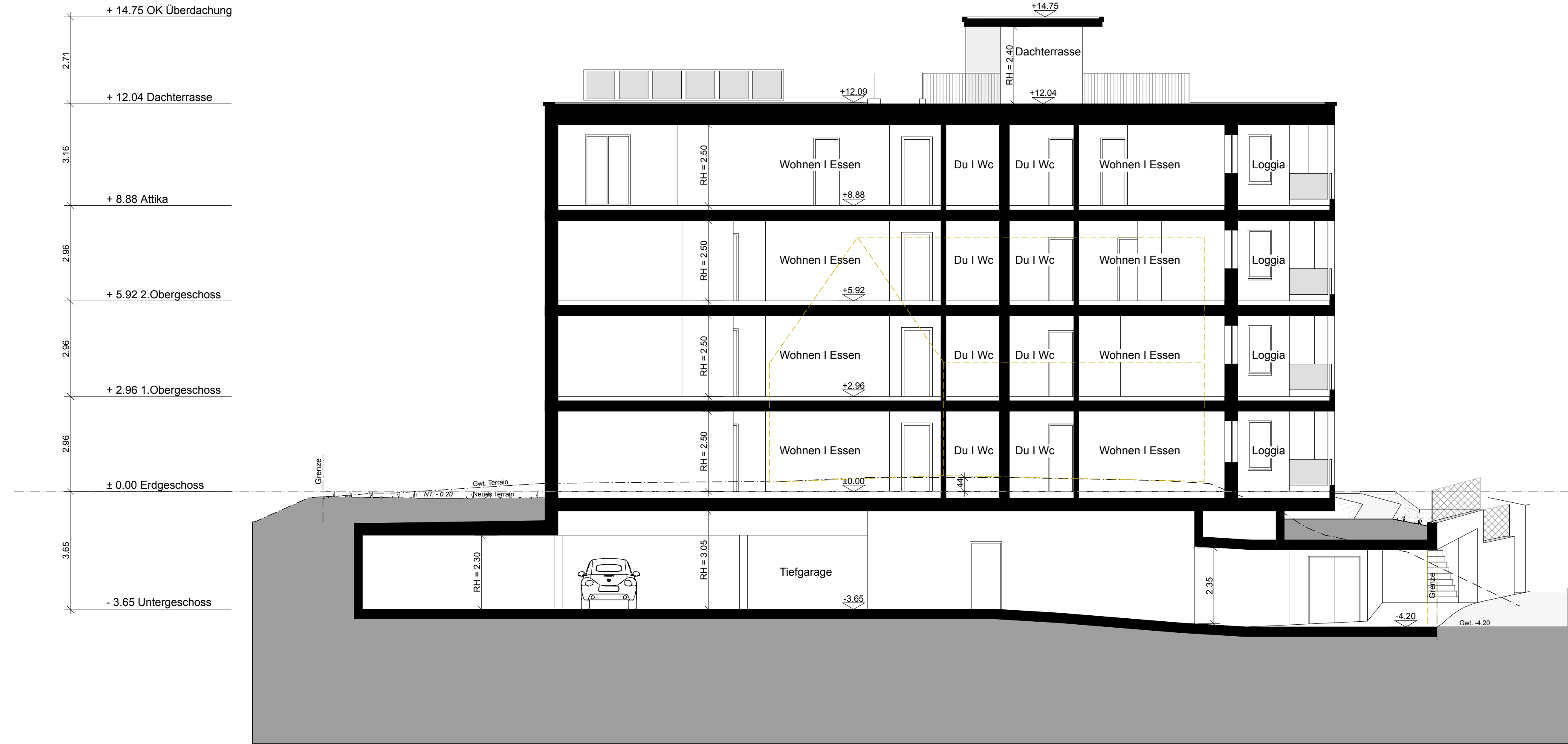
Schnitt 1-1
